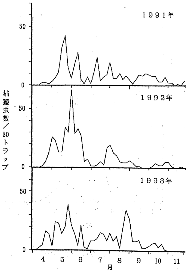
図1 ピットフォールトラップによる成虫の発生消長の年次推移 (三木よかわ C.C.)
