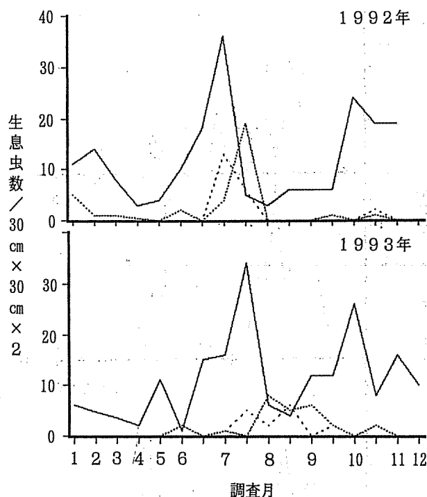
図2 土壌中の齢期別生息密度の比較(千刈 C. C.)
